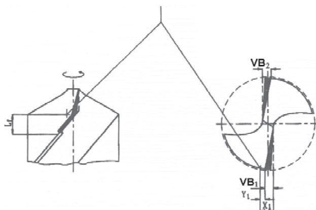
Sl. 3. Značilne oblike obrab pri tazličnih postopkih odrezovanja Fig.3. Characteristic type of wear by different cutting processes
