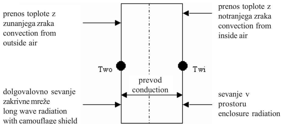
Sl. 2. Energijska bilanca zunanega in notranjega vozlišča stene zavetja Fig. 2. Energy balance for the shelter wall
