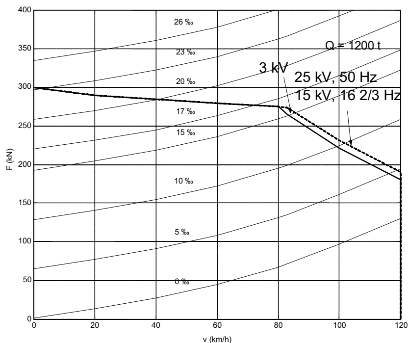
Sl. 3. Vlečna karakteristika lokomotive 6 MW in upori vlaka z maso 1200 t
