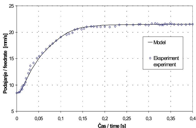
Sl. 4. Primerjava dejanskega in simuliranega podajanja
