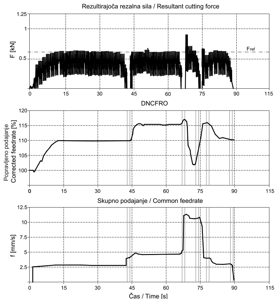
Sl. 12. Preizkus-2: obdelava nepravilnega profila z ločenim optimiranjem rezalnih pogojev in prilagodnim nastavljanjem podajanja
