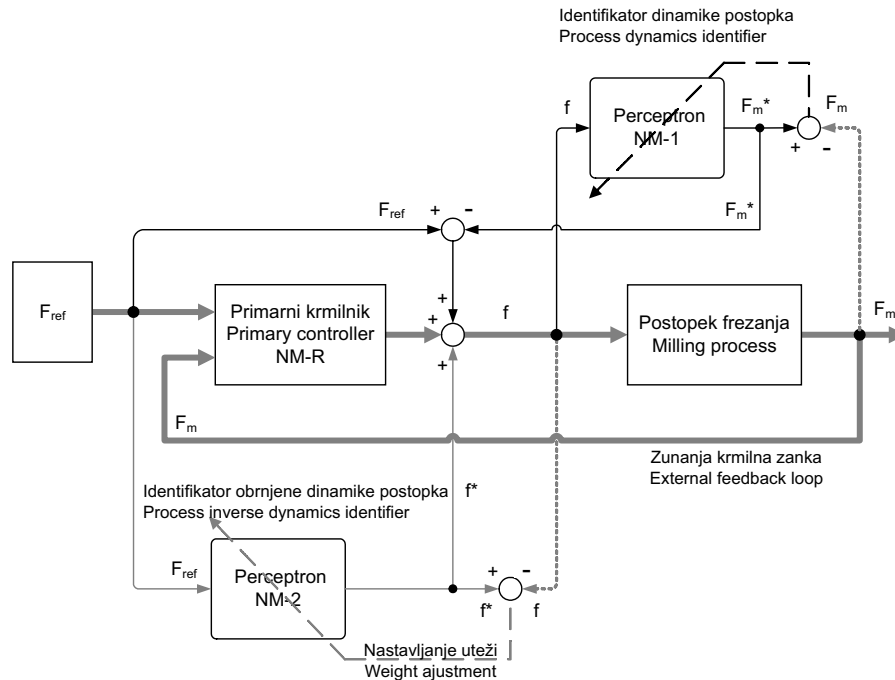
Sl. 2. Usmerjena nevronska krmilna shema (UNKS)
