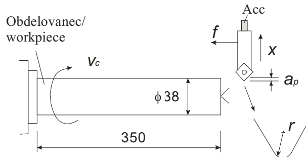
Sl. 10. Testiranje vplivnosti polmera rezalnega orodja ( f -podajanje, v_c -rezalna hitrost, r -polmer rezalnega orodja, Acc-merilnik pospeškov)
