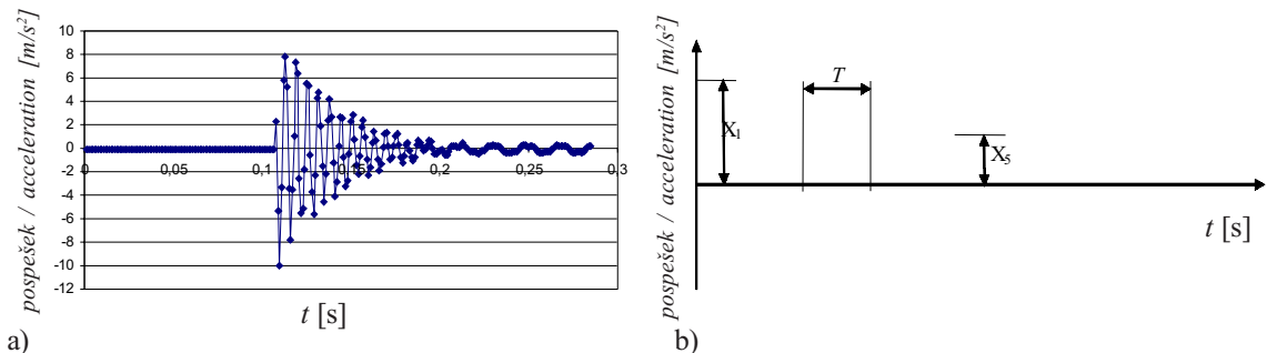
Sl. 9. Rezultati vzbujanja z udarnim kladivom; a) vhodni podatki, b) značilni parametri Fig. 9. Impact hammer testing results; a) input data, b) characteristic parameters
