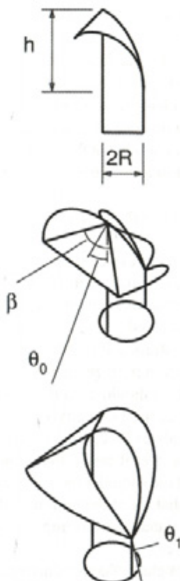
Fig. 5. Parameters of a shoulder
