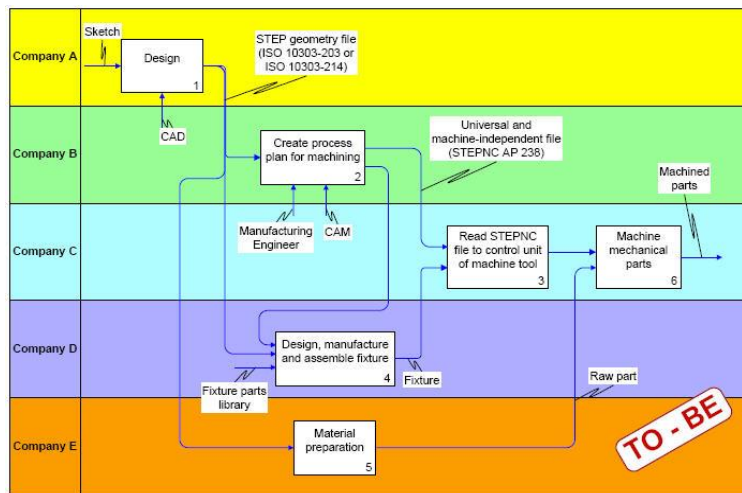
Slika 1. Upravljanje s podatki za obdelavo kot ga predlaga standard STEP-NC
