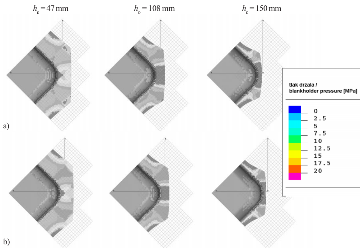
Sl. 4. Porazdelitve tlakov po prirobnici za različne začetne tlake pridrževanja: a) p_d = 3,6 MPa na vseh segmentih ter b) p_d = 3,6 MPa na ravnih delih in p_d = 2,4 MPa v vogalih Fig. 4. Distribution of pressures on the flange for different initial holding pressures: a) p_d = 3.6 MPa on all segments and b) p_d = 3.6 MPa on the straight parts and p_d = 2.4 MPa on the edges
