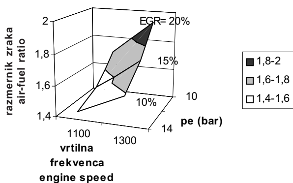
Sl. 4. Izračunani primerjalni razmernik zrak gorivo v sistemu z nizko-tlačnim vračanjem Fig. 4. Predicted equivalent air-fuel ratio with low-pressure EGR
