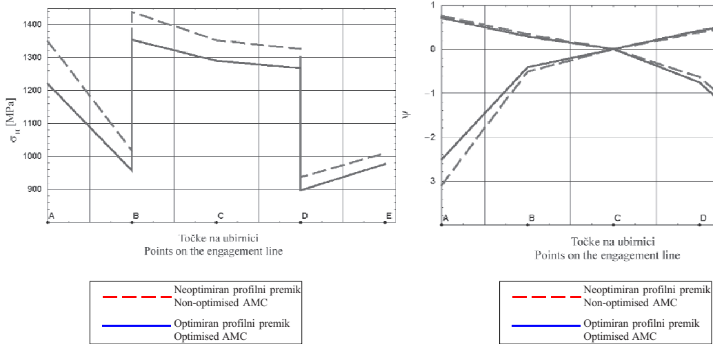
Sl. 8a. Porazdelitev specifičnega drsenja in Hertz-ovega tlaka vzdolž ubirnice Fig. 8a. Specific sliding and Hertz pressure distribution along the path of contact
