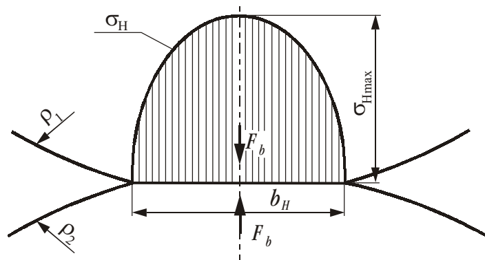
Sl. 4. Hertzova porazdelitev napetosti
